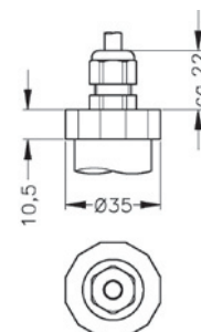
Кабельный ввод
