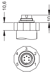
Binder 723 (5-конт.)
