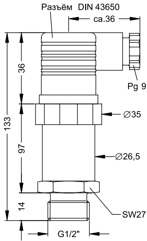
G 1/2" DIN 3852
