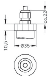
Кабельный ввод
